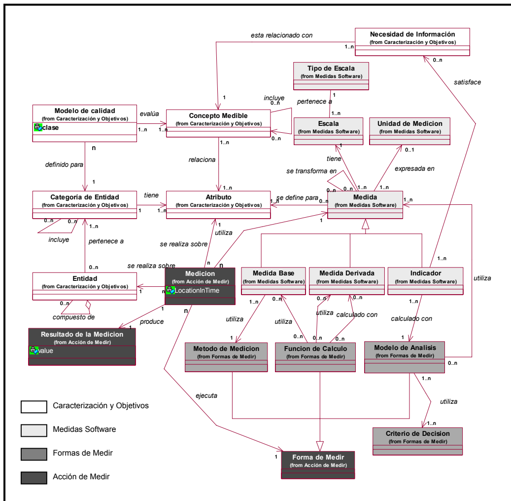
Fig. 2. Metamodelo de Medición del Software
